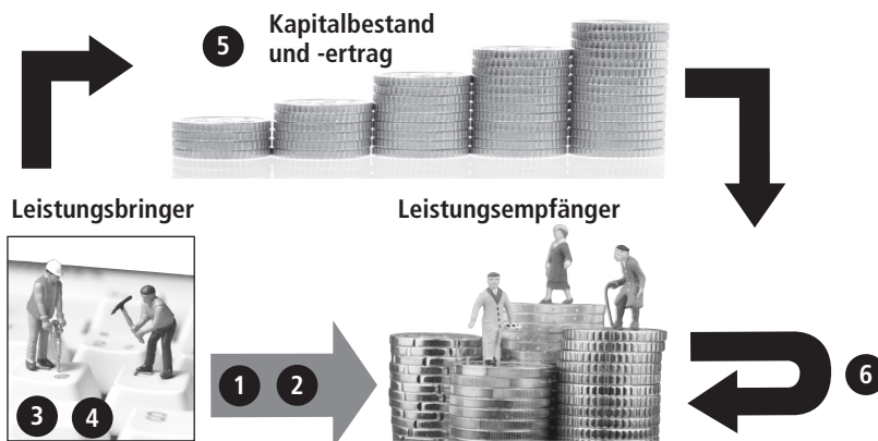
Abbildung 38: Das Verhältnis von Leistungserbringern, Leistungsempfängern und Kapitalbestand
