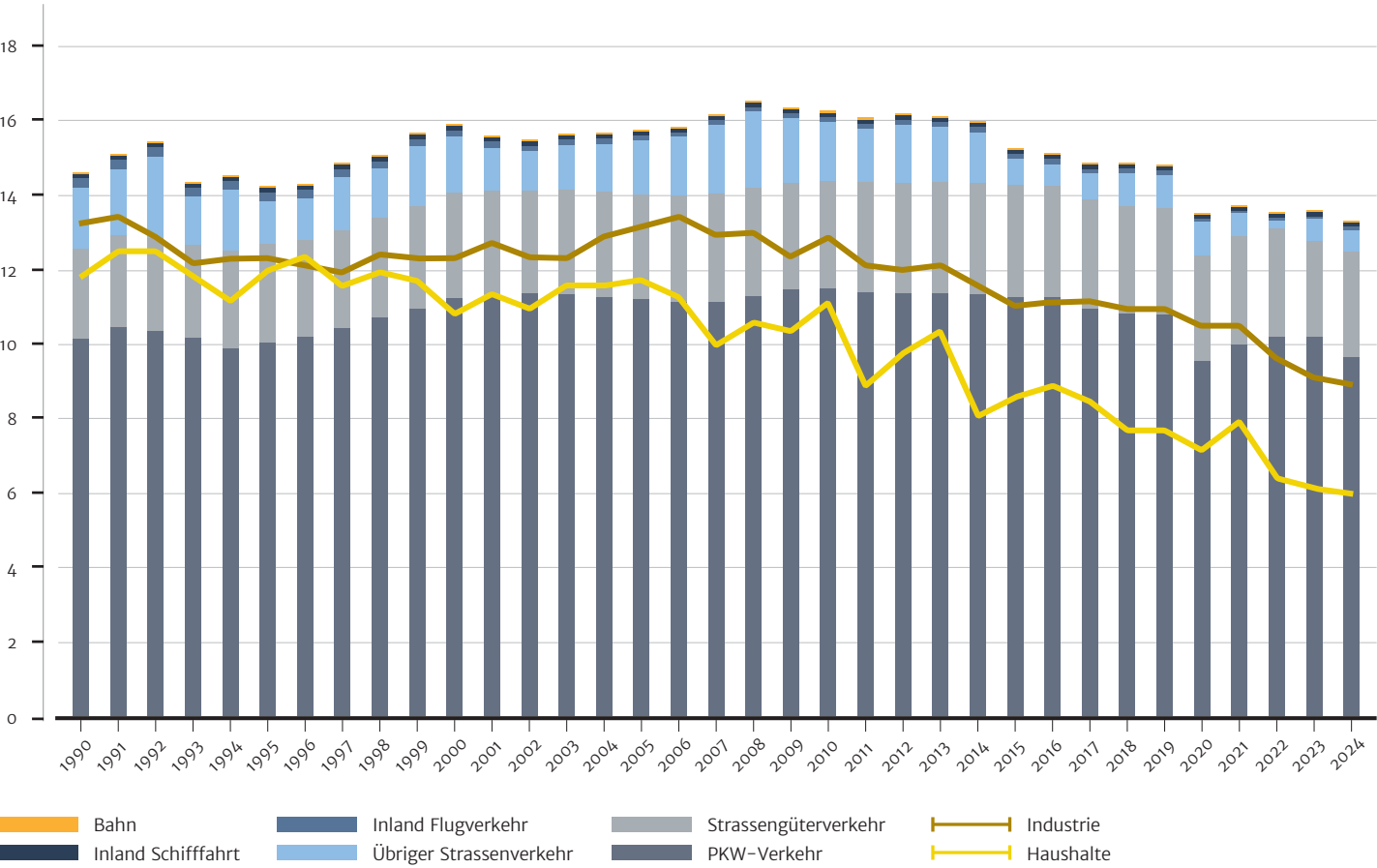
Abbildung 1: Entwicklung der Treibhausgasemissionen im Verkehr der Schweiz nach Verkehrsmittel gegenüber Industrie und Haushalten in Mio. Tonnen CO 2 -Äquivalenten 2024 (BAFU, 2026)
