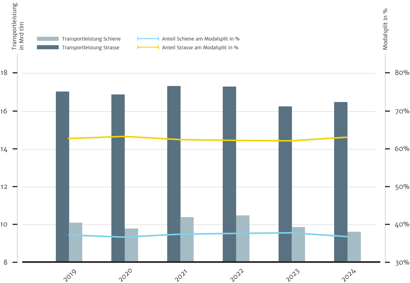
Abbildung 7: Transportleistung Strasse und Schiene und Modalsplit im Güterverkehr der Schweiz (BFS, 2025c)
