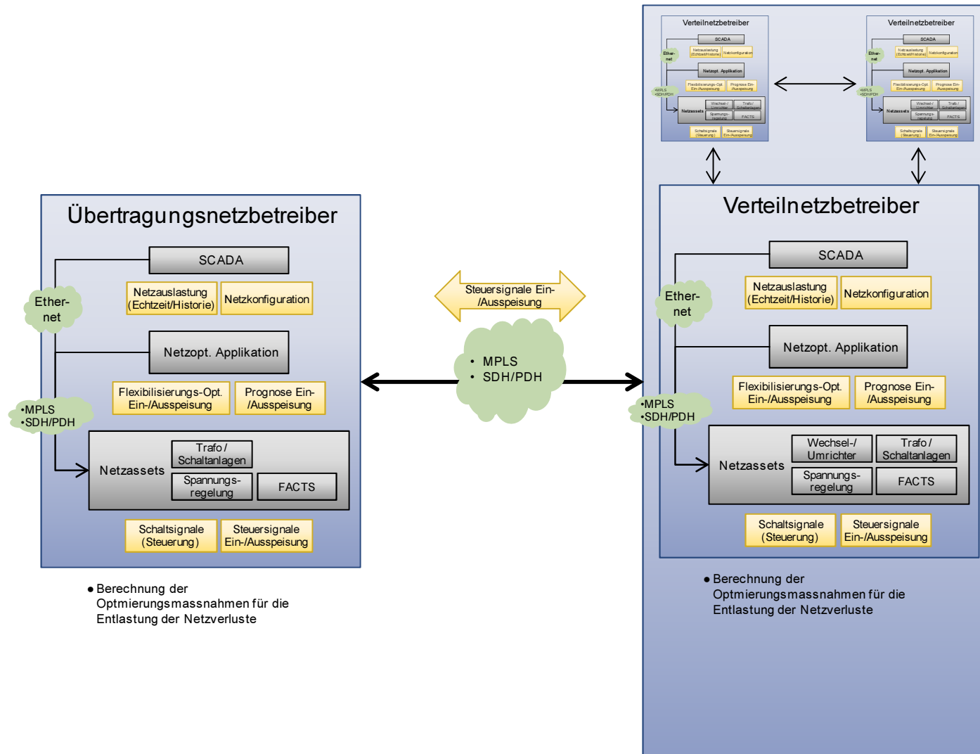
Abbildung 11: Use Case 10 – Reduktion Netzverluste
